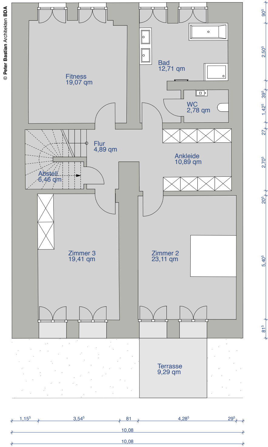
M 1:100
